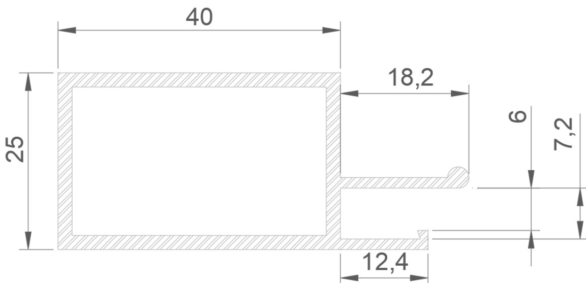
Rysunek 1 Przekrój profilu; wymiary podano w mm
