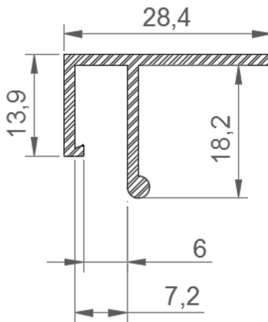
Rysunek 1 Przekrój profilu; wymiary podano w mm
